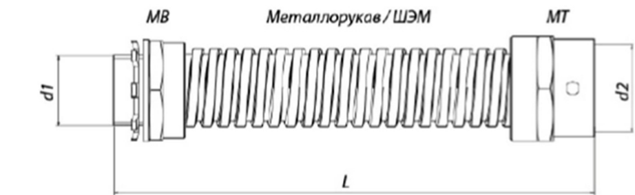
Рисунок 2 - Комплектация. Технические данные.
