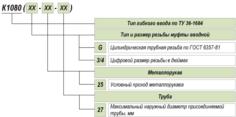
Рисунок 1 - Расшировка обозначения элемента
