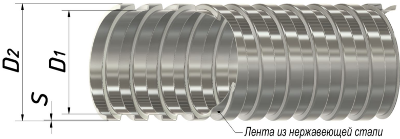
Рисунок 1. Металлорукав типа РЗ-Н
