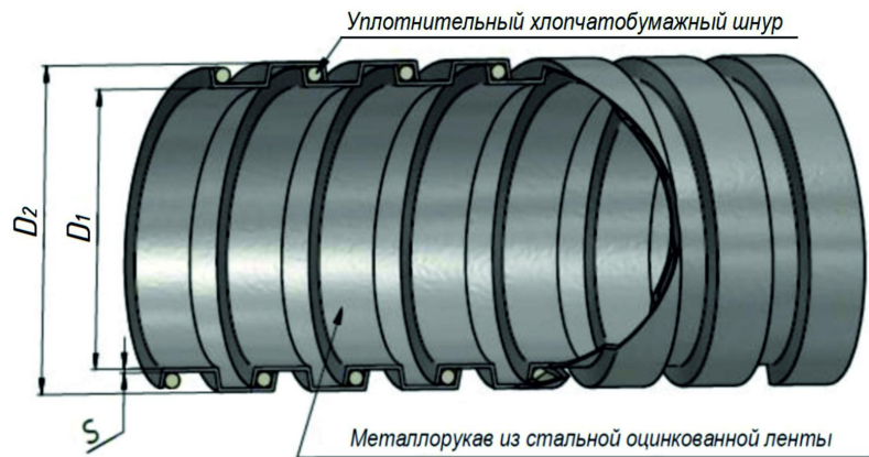
Рисунок 1. Металлорукав типа P3-ЦХ
