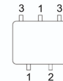
Рисунок 2 — Размещение отверстий для установки фитингов: 1 и 3 - Отверстие Ø26-27 мм; 2 - Отверстие Ø33-34 мм.
