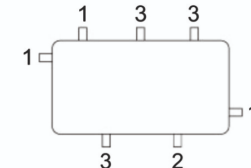
Рисунок 2 — Размещение отверстий для установки фитингов: 1 и 3 - Отверстие Ø26-27 мм; 2 - Отверстие Ø33-34 мм.
