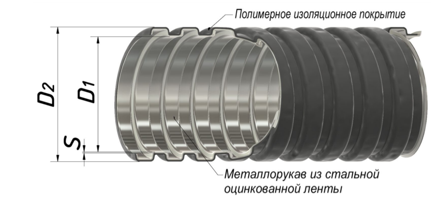
Рисунок 1. Металлорукав типа МРПИ нг морозостойкий
