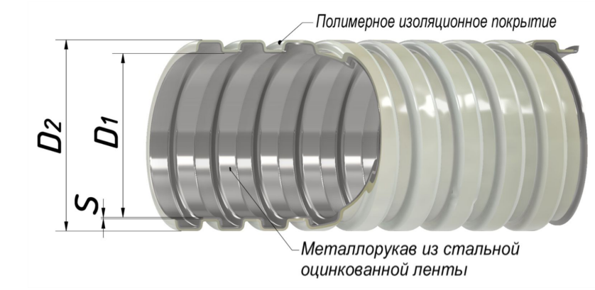
Рисунок 1. Металлорукав типа МРПИ нг серый
