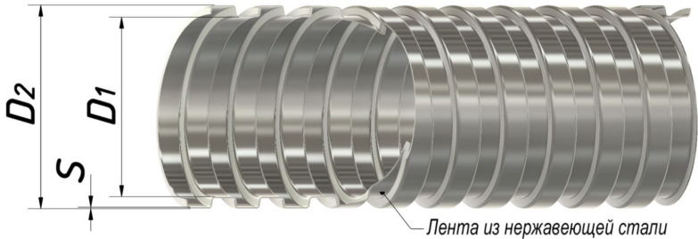
Рисунок 1. Металлорукав типа РЗ-Н
