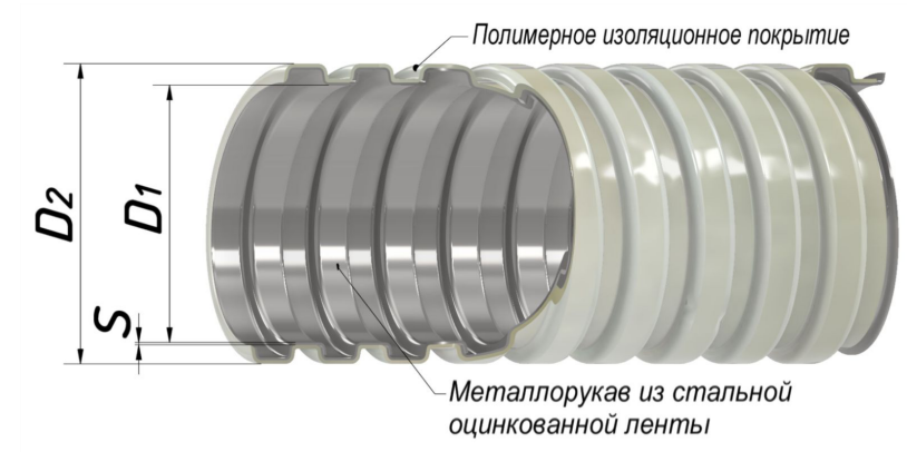
Рисунок 1. Металлорукав типа РЗ-ЦПнг серый
