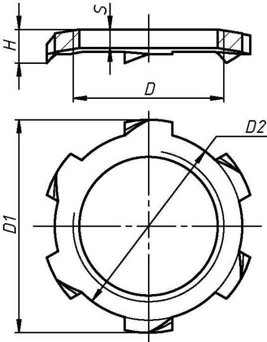
Рисунок 1 - Гайка заземляющая стальная М
