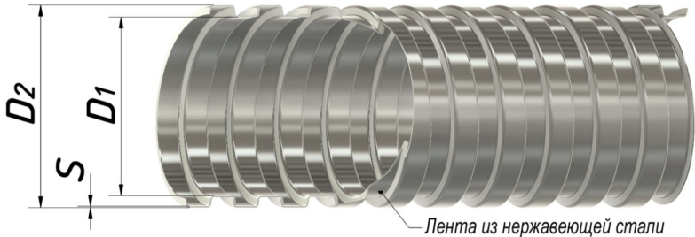
Рисунок 1. Металлорукав типа P3-H
